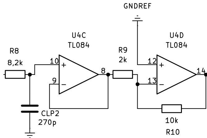
Figura 10: Pasabajos R8–CLP2, seguidor U4C y amplificador inversor U4D. El valor de R9 utilizado es 2,2\text{ k}\Omega ; el rótulo de 2\text{ k}\Omega del esquema no corresponde al valor montado.
