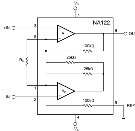
Figura 5: Conexiones básicas y estructura interna del INA122, incluidos los terminales para la resistencia externa R_g . En este diseño no se conecta R_g , por lo que la ganancia nominal es 5. Adaptado de Texas Instruments, p. 1 [25].
