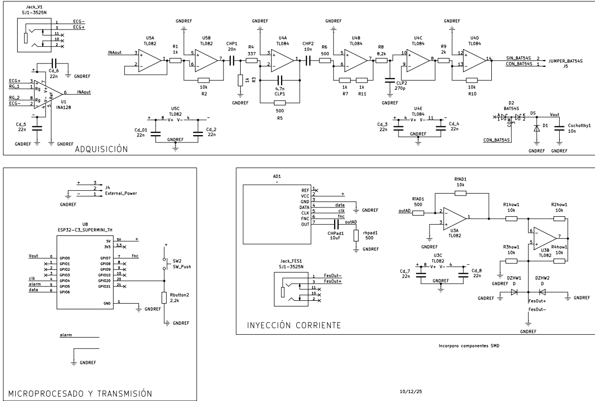
Figura 14: Esquema electrónico general. Los detalles del acondicionamiento se presentan ampliados en la sección de adquisición.
